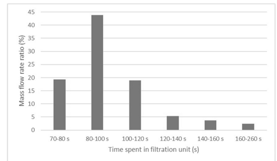
Massenstromverteilung der Verweilzeit im Filter.
