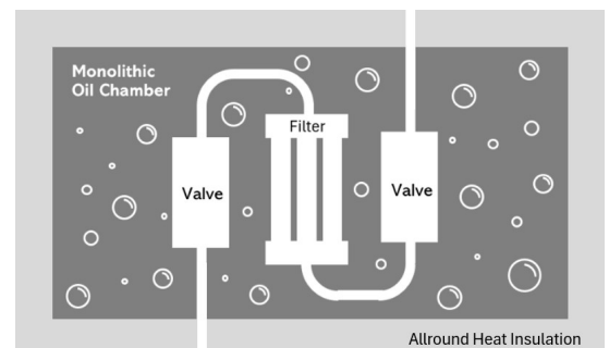
FLUX Monolithic Oil-Chamber-Technologie Gleichmäßige Wärmeverteilung
